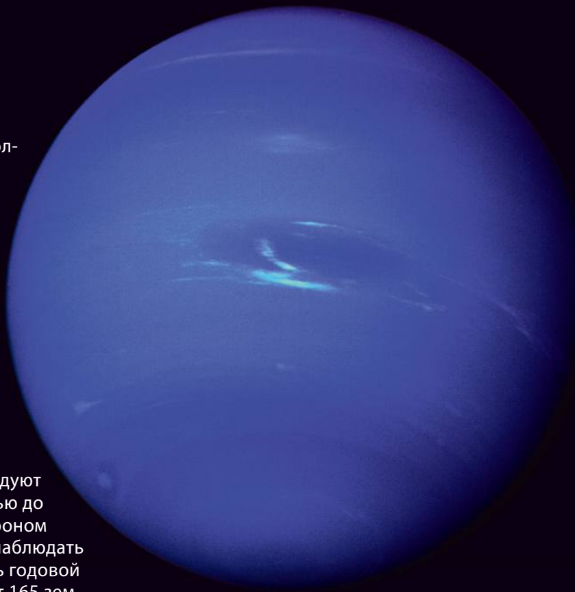
⌘ Фотографии из космоса показывают облачную поверхность Нептуна
