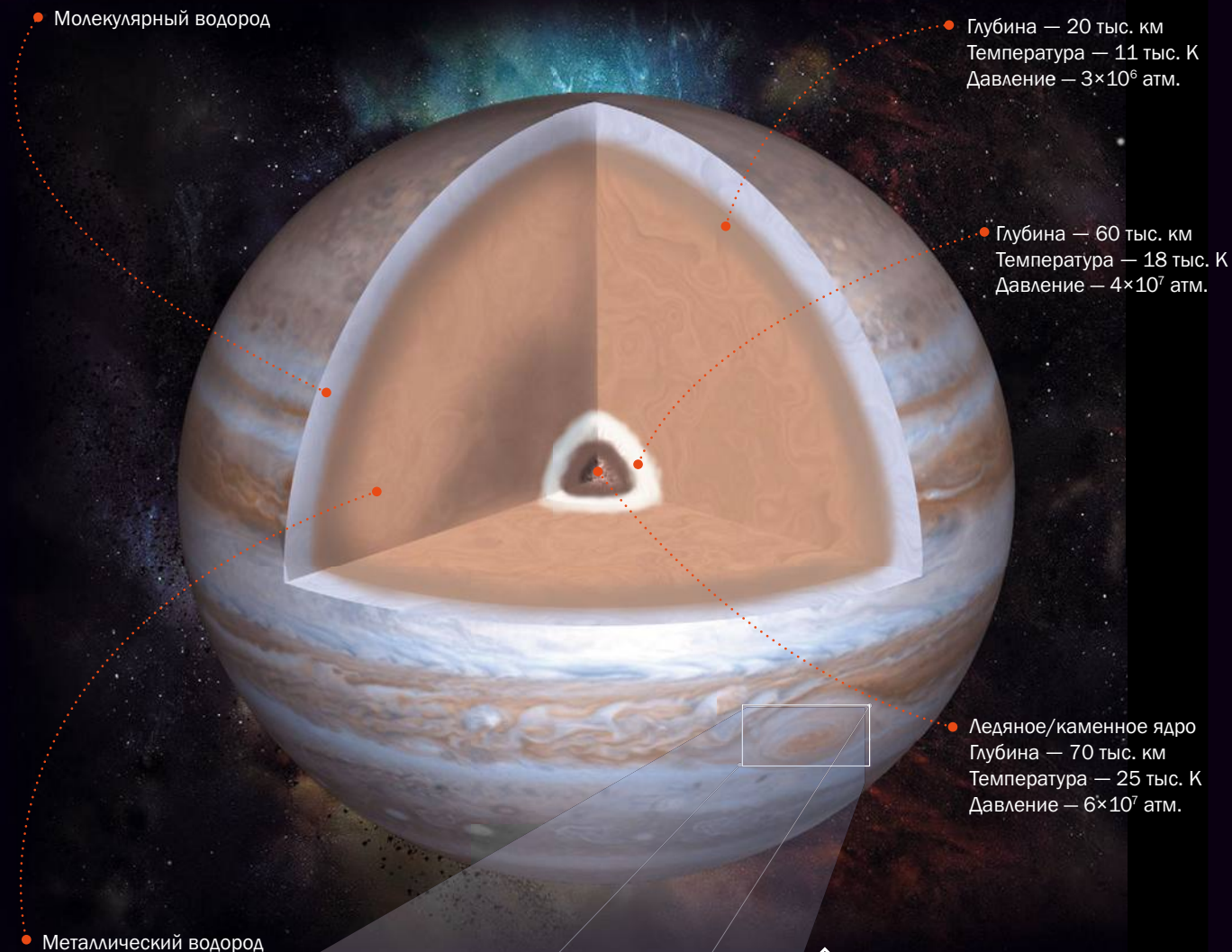
⌘ Строение Юпитера и характеристика атмосферы на разных глубинах
