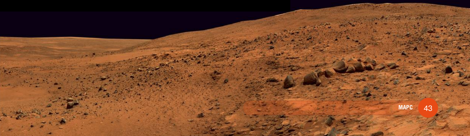
✓ Панорама поверхности Красной планеты, снятая марсоходом «Спирит» 23–28 ноября 2005 года
